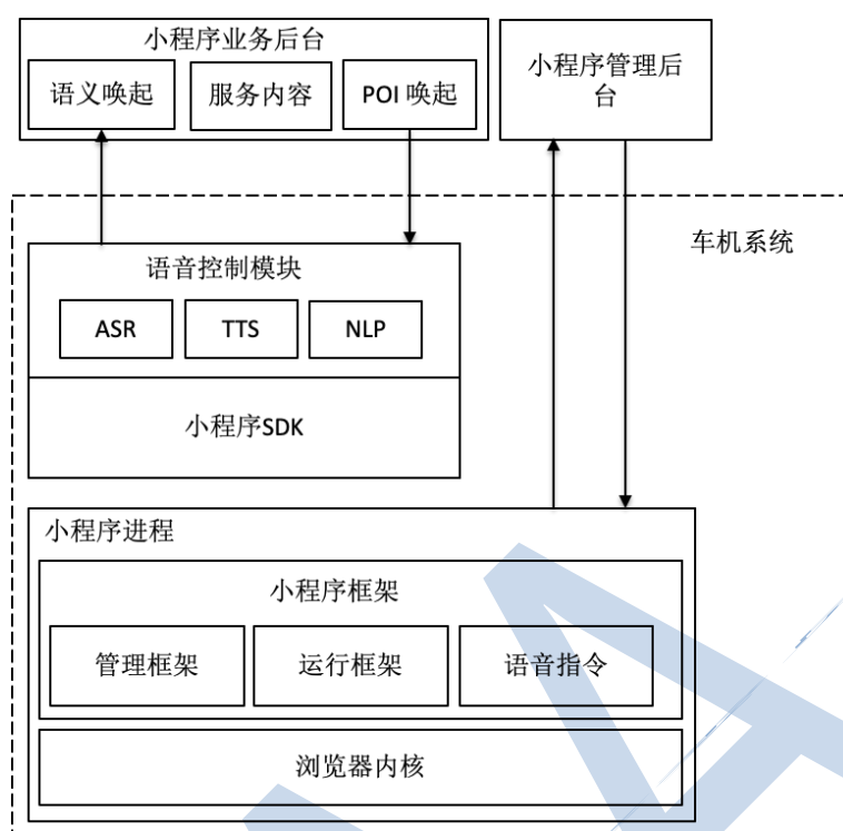
图1 车载小程序框架
